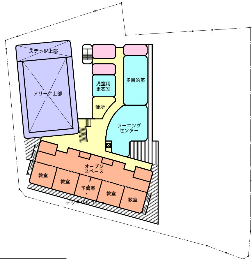
2階平面図
