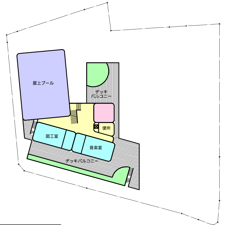
4階平面図
