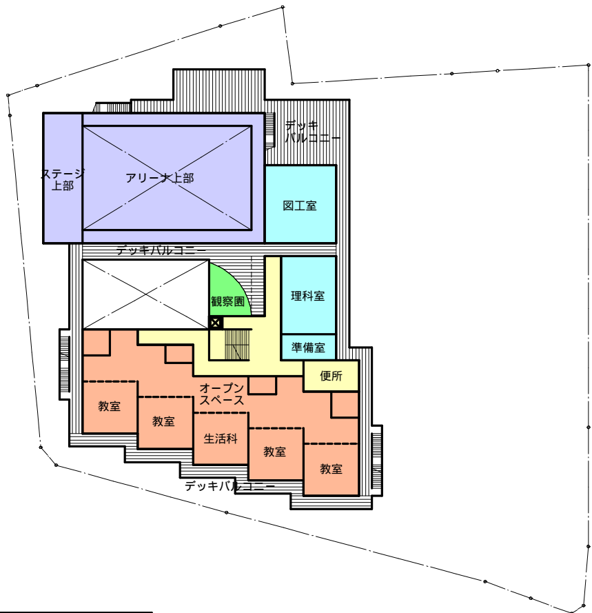
2階平面図
