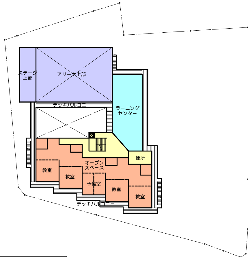
3階平面図
