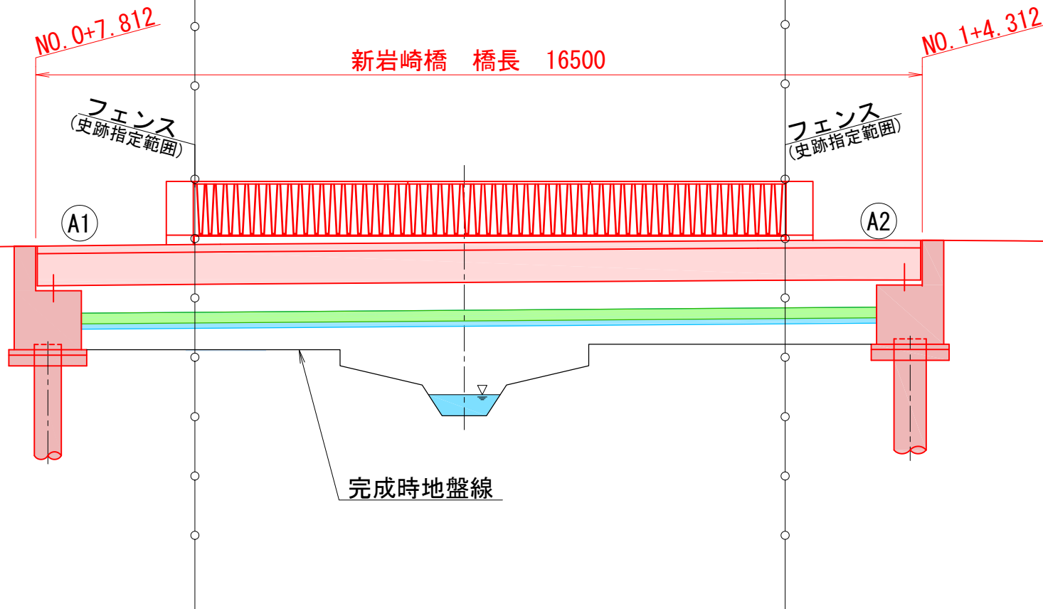
架替後側面図
