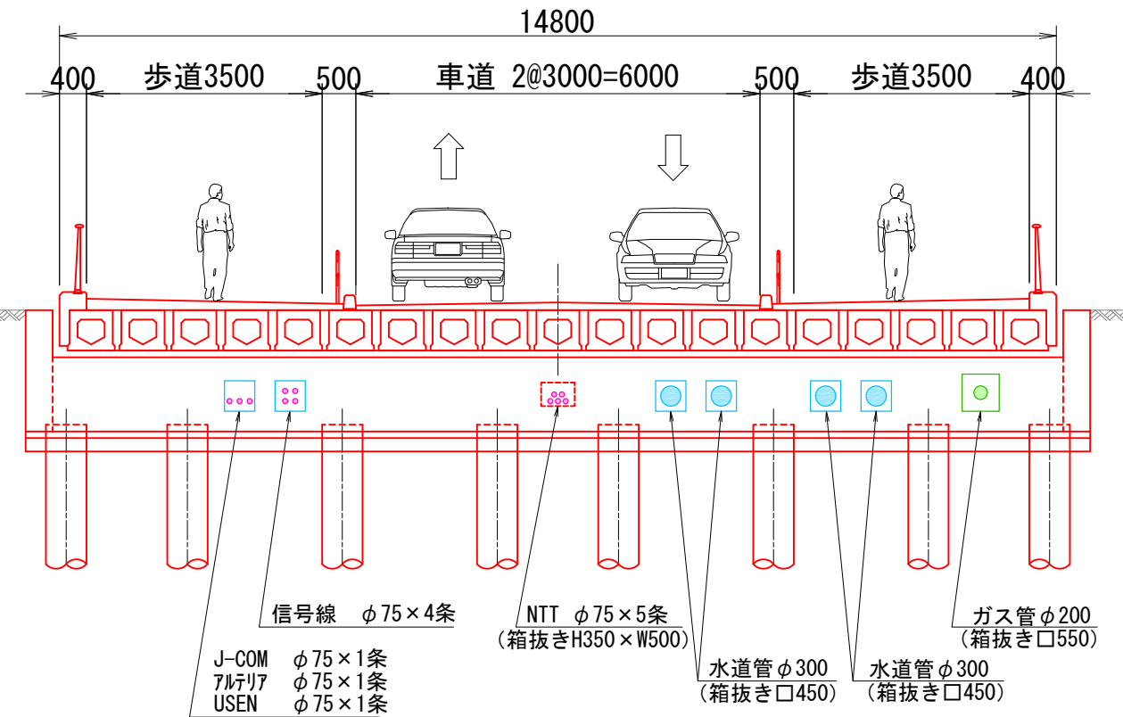
架替後断面図
