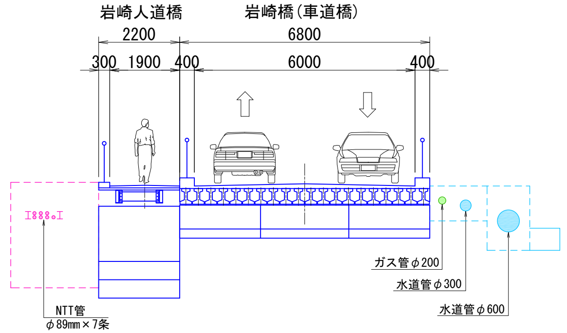
現況断面図
