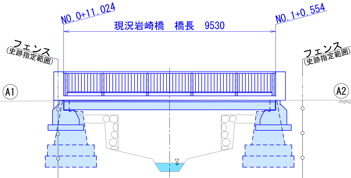
現況側面図
