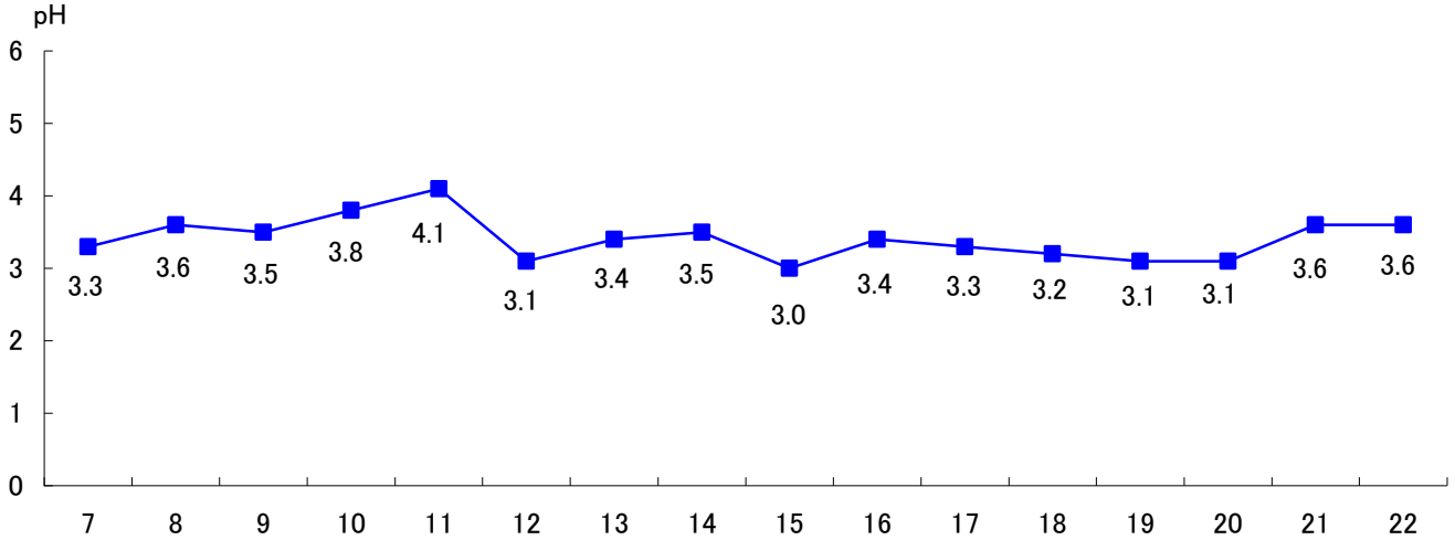
<第3-1-9表> 平成22年度 酸性雨調査結果
