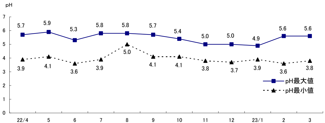
<第3-1-9図> 平成22年度 酸性雨調査結果
