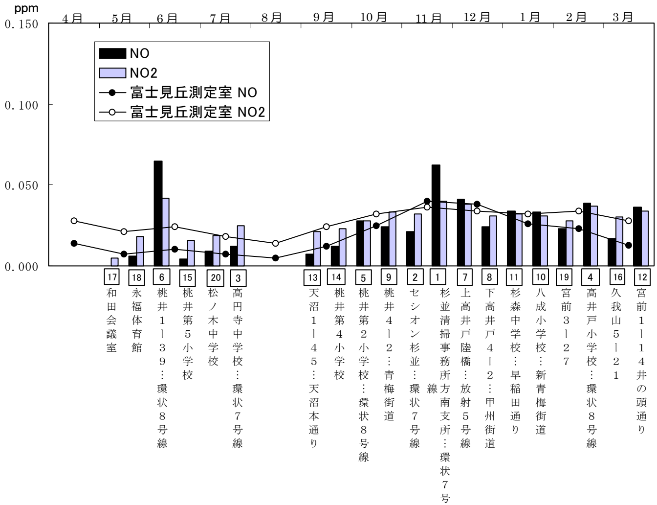
<第3-1-4図> 窒素酸化物連続測定結果（期間平均値）
