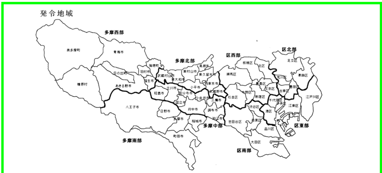
光化学スモッグ発令地域の区分
