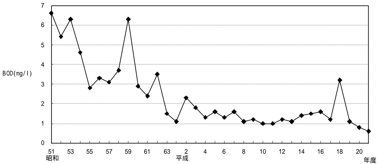
< 第 1 - 3 - 2 図 > 神田川 - 乙女橋での BOD の経年変化
