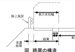
図 路肩の構造
