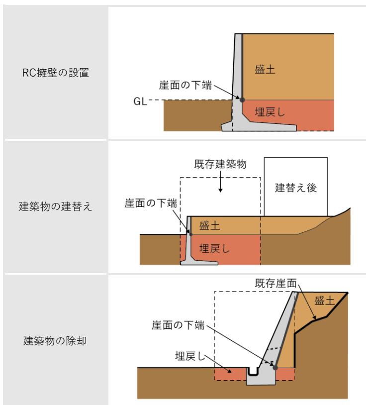
図 1-4 盛土と埋戻し
