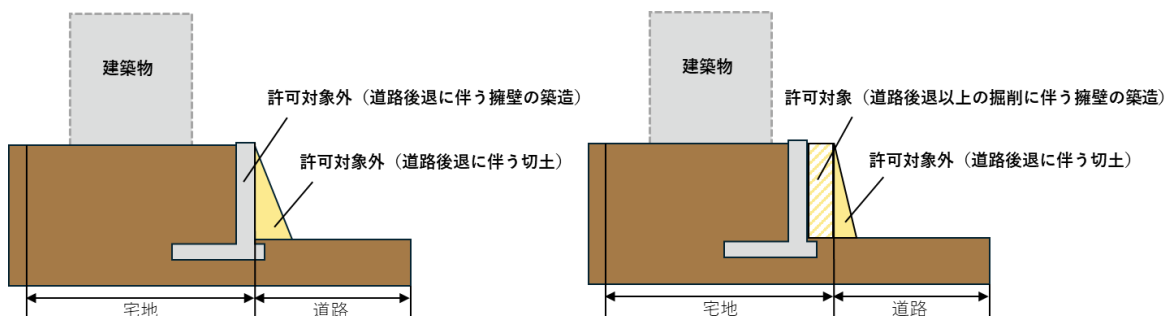
図 1-26 道路後退に伴う造成
