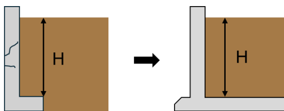
図 1-18 既存擁壁の建て替え
