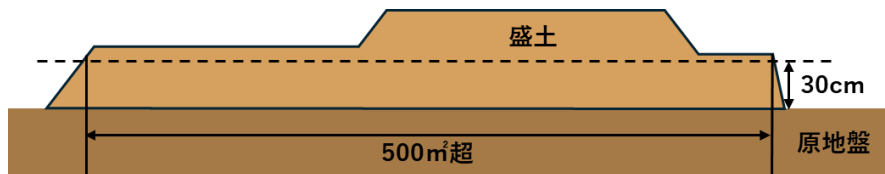
図 1-20 盛土又は切土する土地の面積が 500m 2 超で、盛土又は切土をする前後の地盤面の標高の差が 30cm 超となる場合のイメージ
