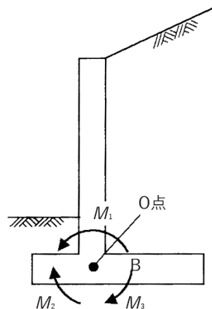
図 3-45 曲げモーメントの関係
