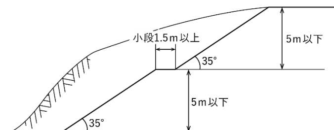
図 3-9 切土法面の形状
