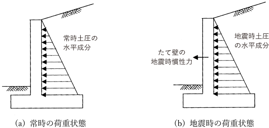
図 3-40 縦壁の断面計算における荷重状態
