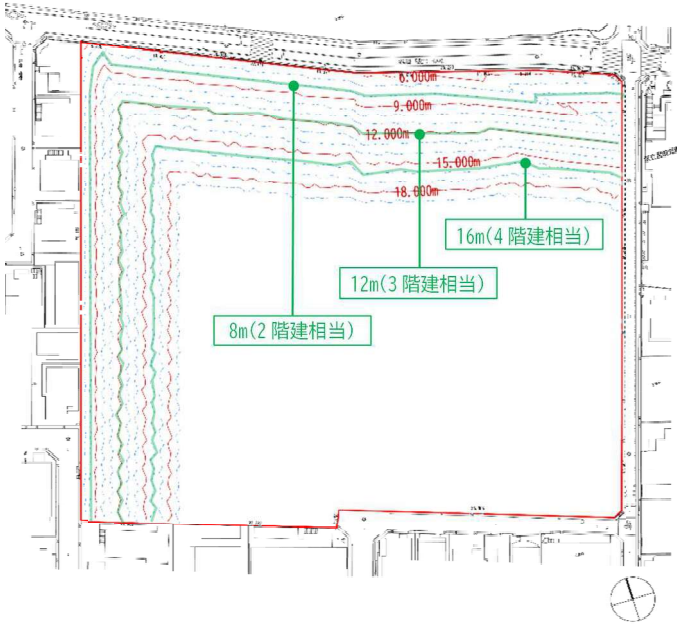
図 1.2.2 日影規制内で建築可能な建物高さ
