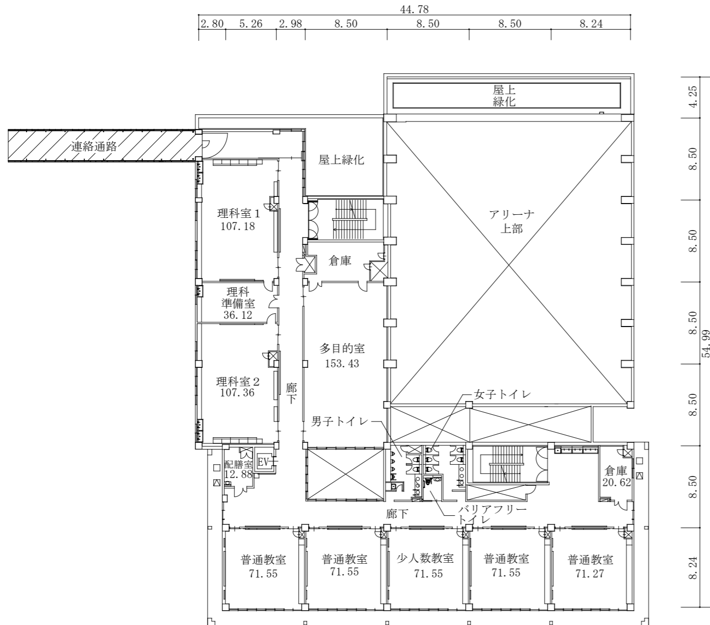
3階平面図
