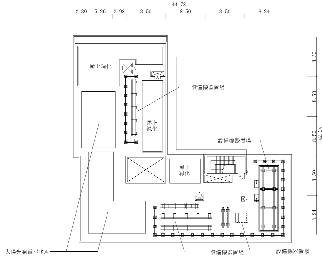
屋上平面図
