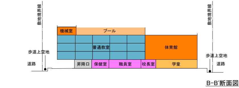
B-B'断面図
