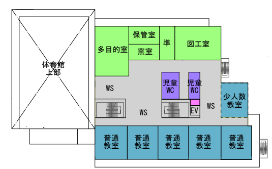
4階平面図
